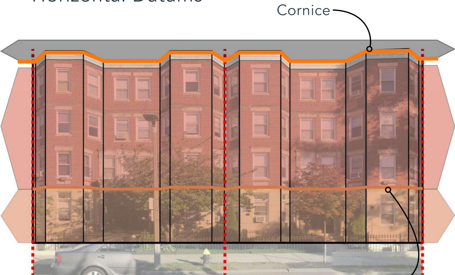
Horizontal Datums
